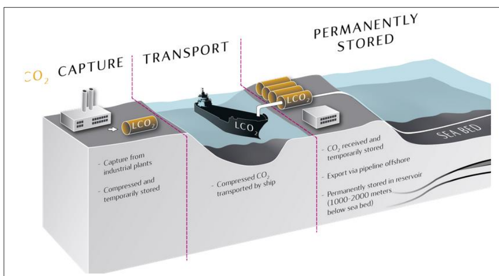
Figura 11. Classico schema di cattura trasporto e stoccaggio di CO 2 (Equinor)
