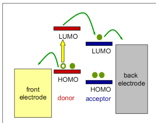
Figura 4. Schema dei livelli energetici e funzionamento di una cella polimero – fullerene
