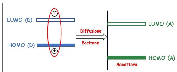
Figura 7: Formazione e diffusione degli eccitoni.
