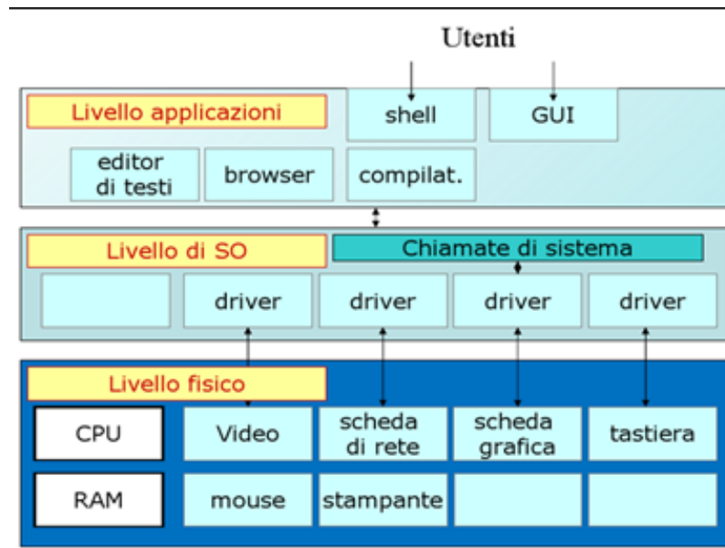
Figura 3. Architettura di un sistema operativo.
