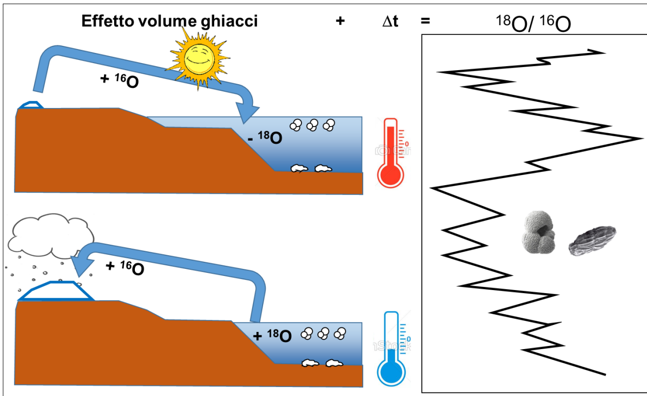
Figura 4. Il cambiamento del ^{18}\text{O}/^{16}\text{O} nel carbonato biogenico marino è connesso non solo a variazioni di temperatura ma anche variazione del volume dei ghiacci continentali. In effetti si ritiene che la variazione nel delta isotopico registrata tra l'ultimo periodo glaciale e l'attuale interglaciale sia riconducibili per circa il 70% al volume dei ghiacci. Il restante 30% è riconducibile alla variazione delle temperature e, regionalmente, a variazioni di salinità.
