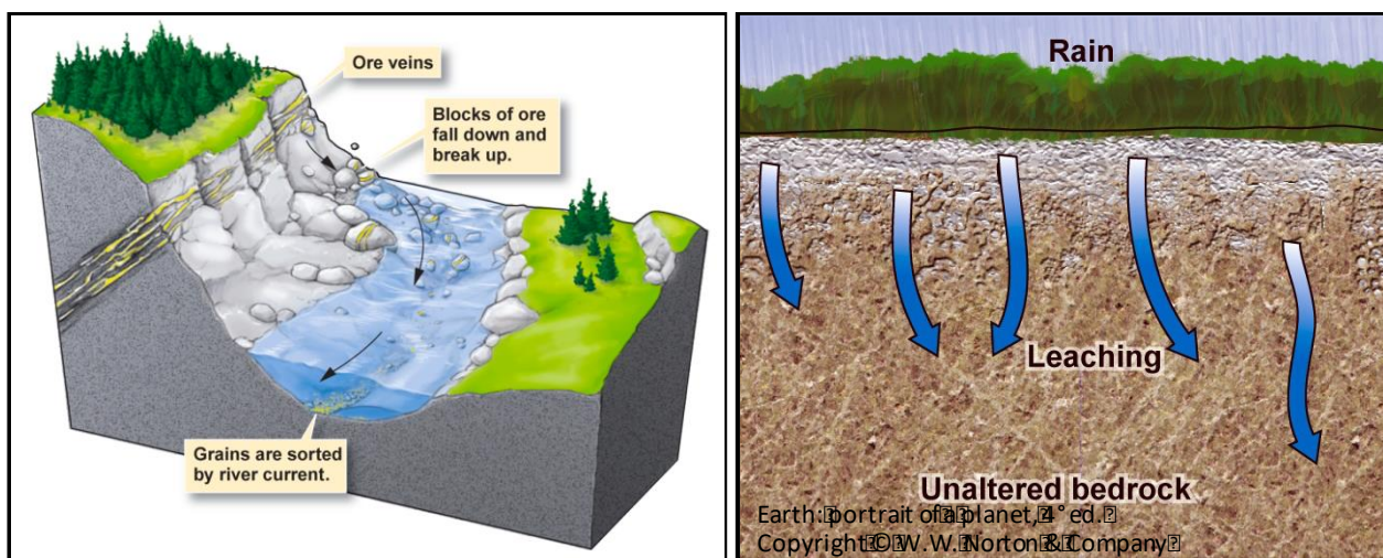
Figura 4. (a sinistra) Modello che mostra come si forma un deposito fluviale di pepite d'oro, per erosione di vene aurifere ipogeniche. (a destra) Processo di alterazione chimica di una roccia silicatica ad opera di acque piovane che penetrano nel suolo. La percolazione di acqua nel sottosuolo dilava la silice e permette l'accumulo residuale degli idrossidi di alluminio.
