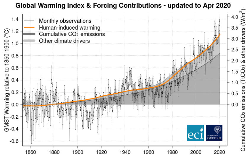
Figura 8. Andamento delle emissioni di CO 2 cumulative e andamento del global warming rispetto al 1850-1900 (riferito come 0.0). Dati Global Warming Index. Oxford.
