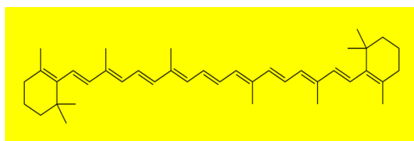
Carotenoidi
