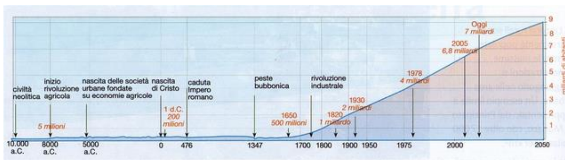
Figura 2. Stima dell'evoluzione della popolazione globale dal 10000 aC sino al 2050.
