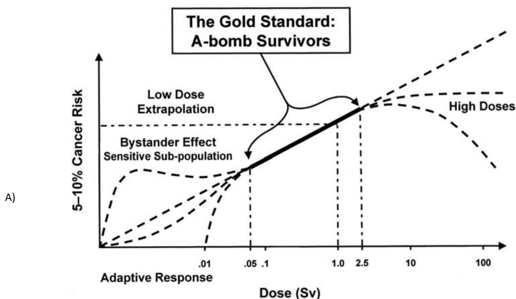
Fig.3: L’LNT model: la linea in grassetto rappresenta i dati sull’incremento di rischio di tumore in funzione della dose ottenuti dagli studi epidemiologici sui sopravvissuti all’atomica di Hiroshima e Nagasaki: alle basse dosi, tale andamento lineare è stato estrapolato linearmente, ossia una relazione lineare è stata assunta valida anche a dosi e ratei di dose bassissimi.
