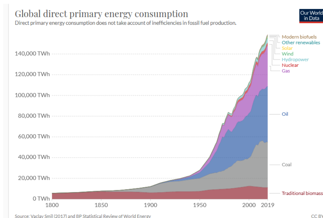
Figura 3. Distribuzione del consumo energetico primario (senza tenere conto delle eventuali inefficienze produttive delle risorse fossili) dal 1800 al 2019. 1Wattora= Wh= 3.6 Kjoule, intesa come un'unità di misura derivata dell'energia, definita come l'energia complessiva fornita qualora una potenza di un watt (W) sia mantenuta per un'ora (h). TWh=10 12 wattora nel tempo. (Dati tratti da BP statistical Review of World Energy 2017).
