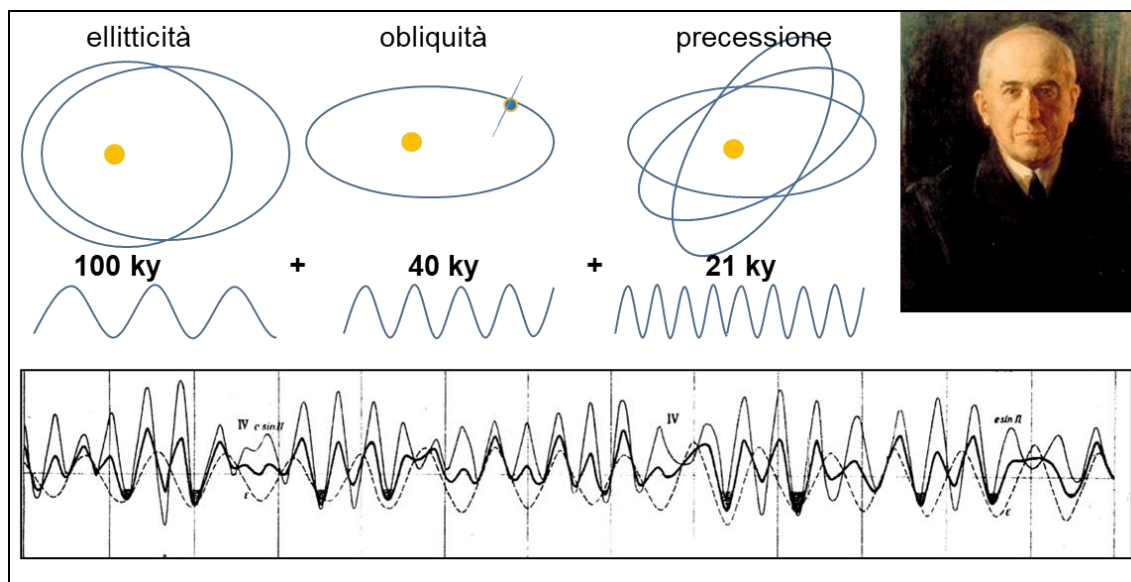
Figura 2. Dalla combinazione dei moti millenari si ottengono le variazioni della insolazione solare alle diverse latitudini nel tempo. Per Milankovitch sono cruciali i valori dell'insolazione estiva nell'emisfero boreale a circa 65°N di latitudine. Si tratta di quelle regioni, occupate da continenti, che risultano rispettivamente occupate o libere da calotte nei periodi glaciali e interglaciali. Bassi valori di insolazione estiva determinano uno scioglimento solo parziale delle nevi, innescando reazioni di feed-back legate all'aumento dell'albedo (riflettanza complessiva del Pianeta).
