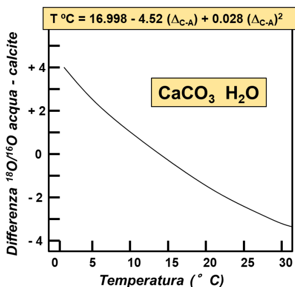
Figura 3. La composizione isotopica del carbonato che cristallizza in acqua è in relazione con quello dell'acqua stessa e con la temperatura: al diminuire della temperatura, il suo rapporto ^{18}\text{O}/^{16}\text{O} sarà via via più distante da quello dell'acqua.
