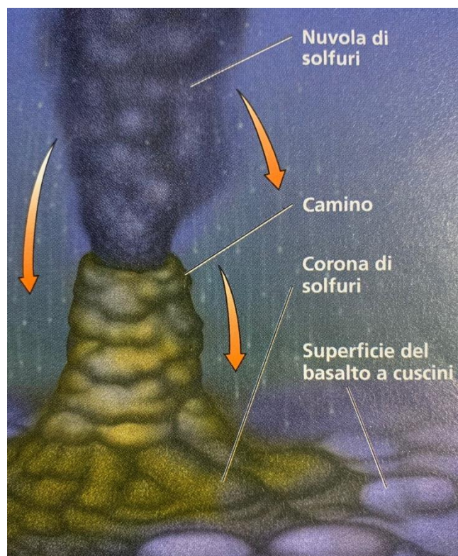
Figura 3. (a sinistra) Rappresentazione schematica di una camera magmatica che, raffreddando lentamente, permette la cristallizzazione di solfuri metallici. (a destra) Concrezioni a forma di "camino" formatesi al di sopra del fondale oceanico in corrispondenza di emissioni sottomarine di fluidi idrotermali.
