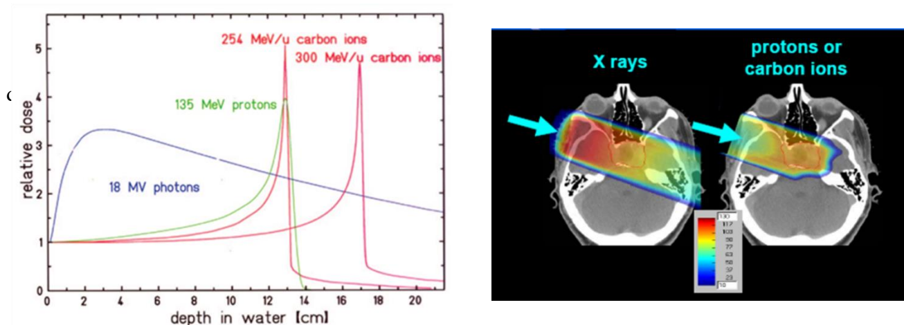
Fig. 5. A sinistral i profili di dose dei fotoni comunemente usati in RT e quelli delle particelle (protoni e ioni carbonio,) usati in adroterapia; a destra un piano di trattamento mediante il quale il fisico medico mediante opportuni programmi computerizzati definisce i contorni di dose ai vari organi/tumori
