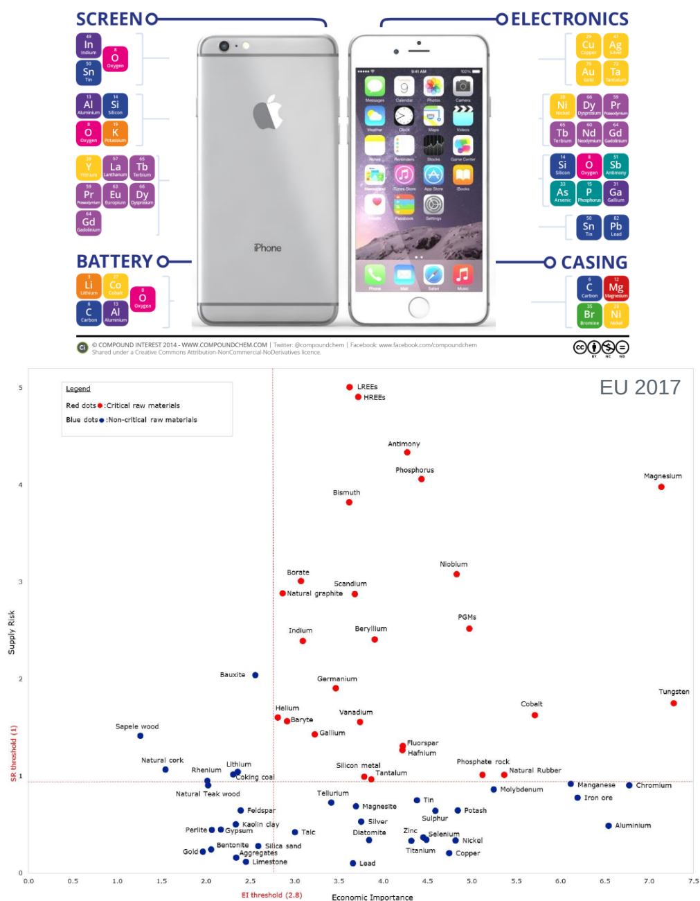
Figura 1.- (in alto) Elementi in uso in un moderno smartphone. (in basso) Distribuzione degli elementi chimici e delle materie prime di interesse economico sul diagramma di “criticità” (Importanza economica vs. rischio di approvvigionamento). Sono evidenziati in rosso gli elementi e le materie prime che, presentando alta importanza economica ed alto rischio di approvvigionamento, sono definiti “critici” (Commissione Europea 2017).
