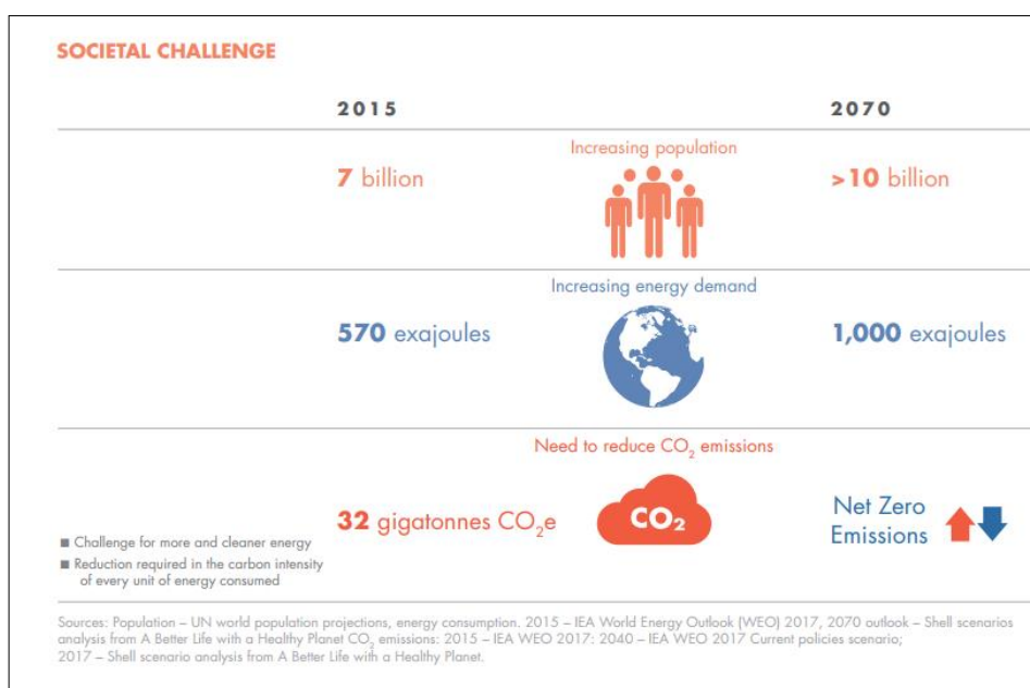
Figura 10. Stime e proiezioni di crescita di energia, popolazione ed emissioni di CO 2 (dati IEA World Energy Outlook 2017)
