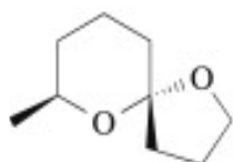
(5R,7S)-7-metil-1,6-diossapro[4.5]decano
