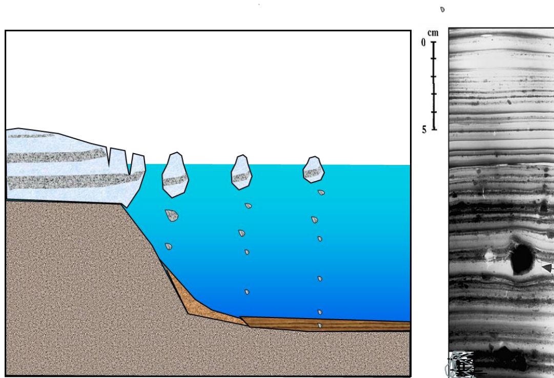
Figura 7. Gli eventi di Heinrich sono in relazione con la presenza, in depositi dei fondali dell'Oceano Atlantico, di detriti di origine glaciale rilasciati da grandi iceberg prodotti dalla destabilizzazione delle calotte continentali.
