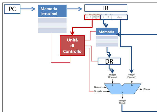
Figura 4. Rappresentazione schematica di una CPU
