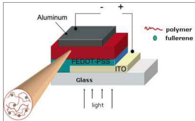
Figura 3. Architettura di una semplice cella polimerica solare dove lo strato attivo viene depositato secondo il concetto della bulk heterojunction.
