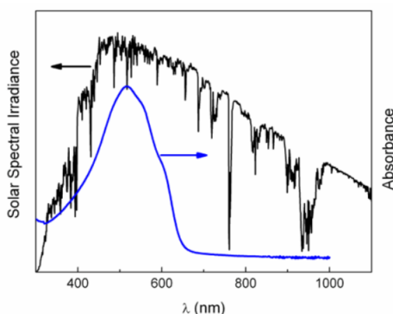
Figura 5: Spettro solare (in nero) e assorbimento del P3HT (in blu)
