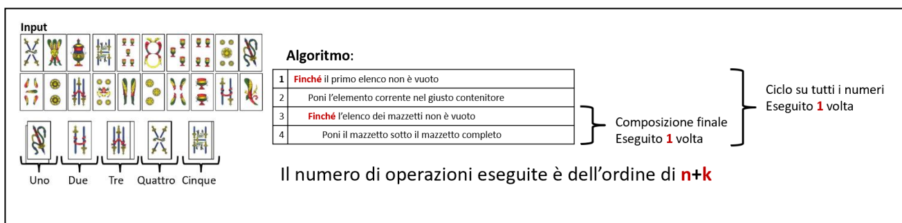
Figura 9. Algoritmo di ordinamento Counting Sort.
