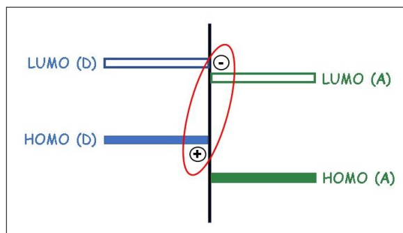
Figura 8. Trasferimento di carica dal donore all'accettore
