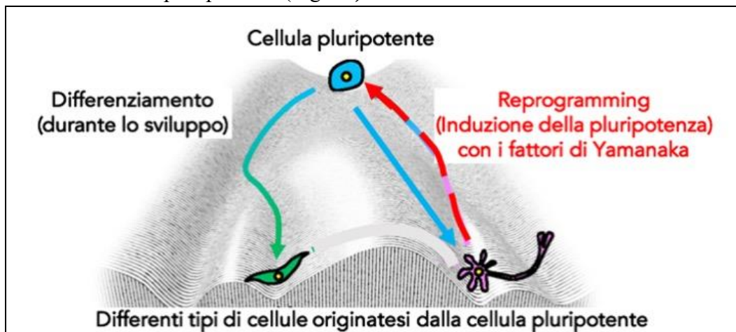
Figura 10. Concetto di riprogrammazione cellulare utilizzando il modello di Waddington (modificato da Takahashi and Yamanaka, 2013).
