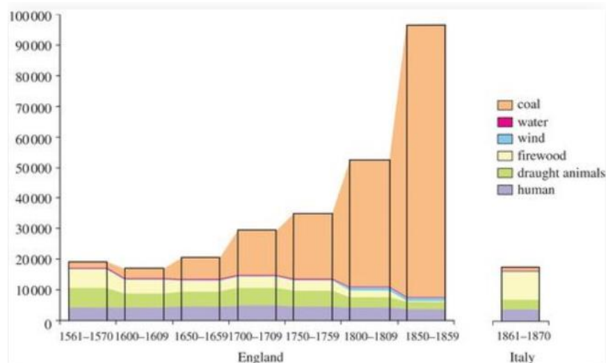
Figura 5. Distribuzione delle risorse energetiche a partire dal rinascimento sino alla rivoluzione industriale. (Dati tratti da Energy and the English industrial Revolution . Wrigley, 2013. Phil Trans of the Royal Society A )
