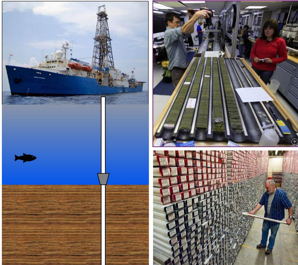
Figura 5. Le carote di sedimenti recuperate in mare profondo nel corso delle campagne oceanografiche vengono sezionate, descritte e campionate per gli studi successivi già a bordo. Dopo vengono conservate (in basso a destra il sito di stoccaggio di Brema, in Germania) in quanto costituiscono un fondamentale archivio di informazioni riguardanti l'evoluzione climatica della Terra nel corso di milioni di anni.
