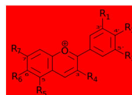
Antocianidine
