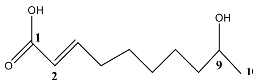
9-idrossi-trans-2-decenoico
