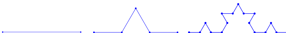
Figura 2. Passi 0, 1, 2 per la costruzione della curva di von Koch
