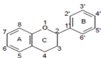
nucleo flavanico
