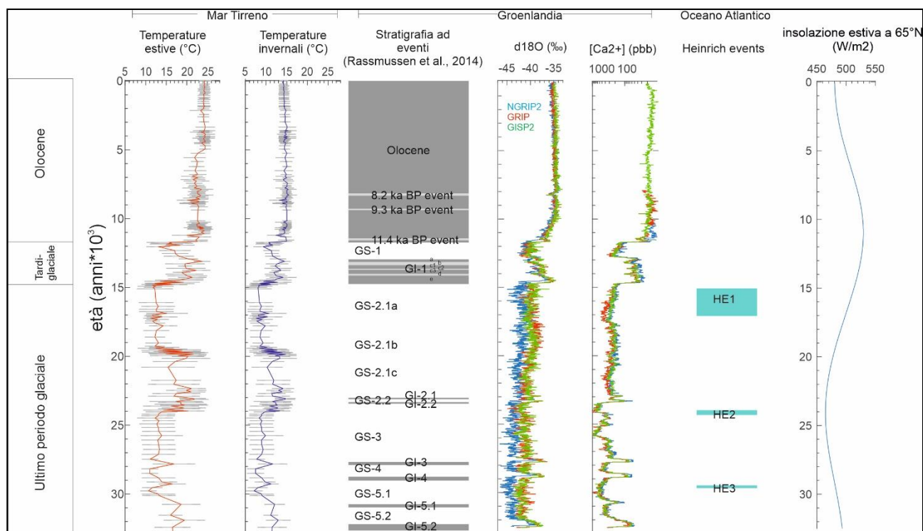
Figura 8. Ricostruzione delle SST estive e invernali del Mar Tirreno ottenute da una Carota recuperata nel Golfo di Salerno. Le barre grigie orizzontali rappresentano l'incertezza associata alla ricostruzione. La ricostruzione è messa in confronto con il record isotopico e geochimico delle carote di Ghiaccio della Groenlandia e i cicli interstediale-stadiale di Rasmussen et al. (2014), la cronologia degli eventi di Heinrich dell'Oceano Atlantico settentrionale e con i valori della insolazione estiva a 65°N di latitudine (dati estratti da Laskar et al., 2004)
