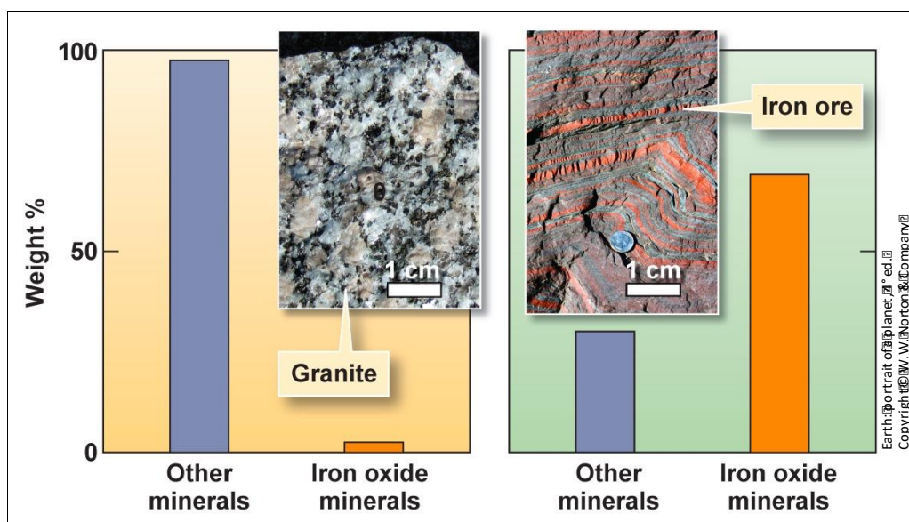
Figura 2. Rappresentazione grafica della differenza tra una roccia “normale (es. un granito), ed un giacimento di ferro. Il granito contiene minerali di ferro (Iron oxide minerals) in quantità troppo bassa affinché possano essere recuperati in maniera economicamente vantaggiosa. Un giacimento di ferro (schema a destra) deve contenere almeno il 60% in peso di minerali di ferro.
