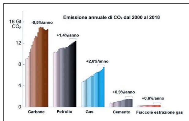
Figura 9. Emissione annuale di CO 2 dal 2000 al 2018 per diverse fonti energetiche. ( Global Carbon Project / L.Bignami)
