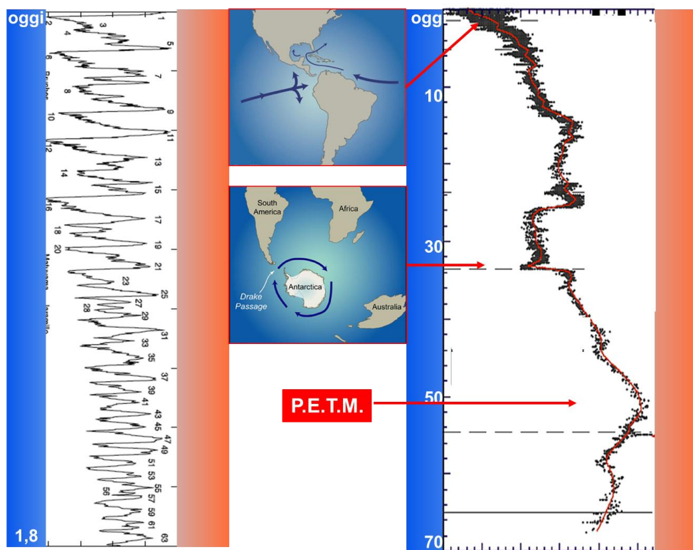
Figura 6. Sulla sinistra il dettaglio dei cicli glaciali degli ultimi 1,8 milioni di anni. Sulla destra le variazioni del Cenozoico con indicati i tre maggiori eventi climatici: il massimo termico della transizione Paleocene-Eocene, l'inizio delle glaciazioni antartiche e l'inizio delle glaciazioni artiche.
