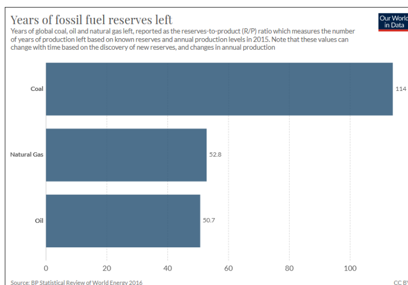
Figura 7. Disponibilità di riserve energetiche fossili attualmente disponibili. Dati ottenuti da BP statistical review of world Energy 2016
