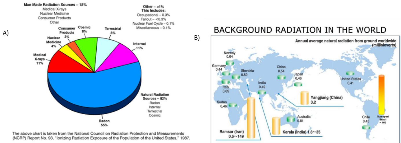
Fig. 1. A) Contributo di varie fonti all'esposizione umana; B) Esistenza di regioni dove la radiazione di fondo è estremamente più alta della media.
