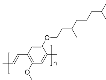
a) MDMO-PPV
