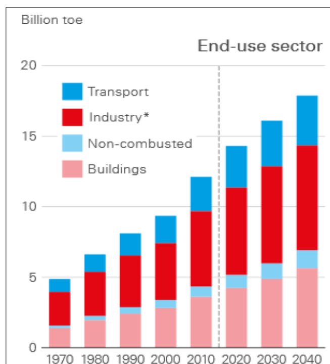
Figura 4. Utilizzo energetico per settori globali (source BP statistical review of World Energy, 2019)
