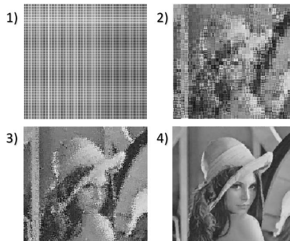
Figura 5. Il processo di decodifica frattale.
