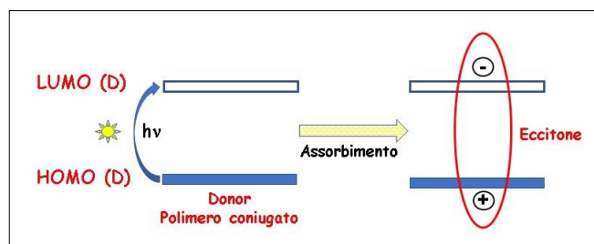
Figura 6. Assorbimento di un fotone e promozione di un elettrone del donatore dall'HOMO al LUMO.
