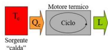
a) Motore termico che non rispetta il Secondo Principio della Termodinamica
